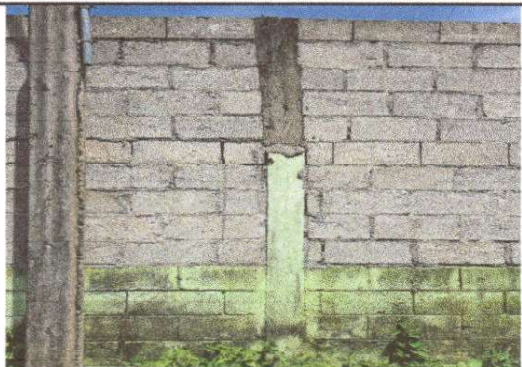
Foto 1: Reparación de muro perimetral, debido a que no existe un refuerzo para sostener el muro y corre el riesgo de caer.
